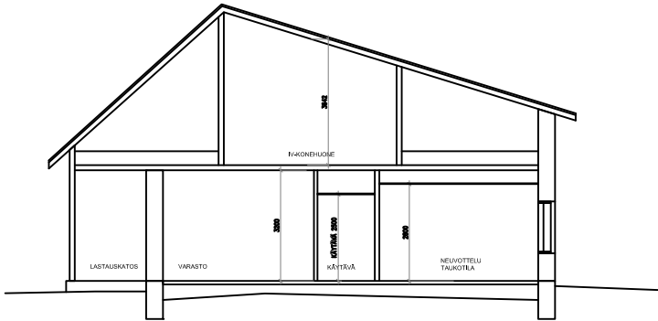
leikkaus c
