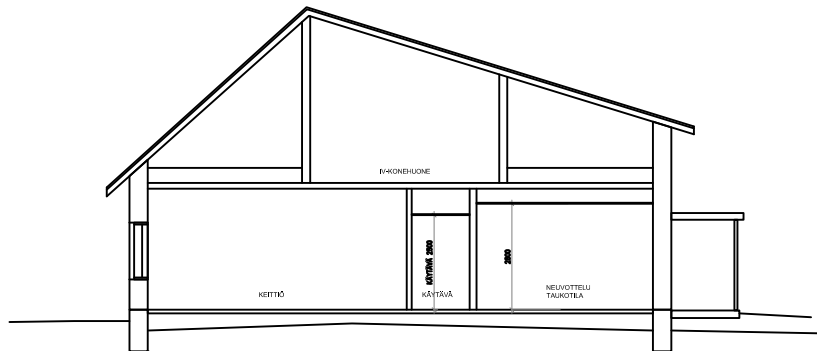
leikkaus b
